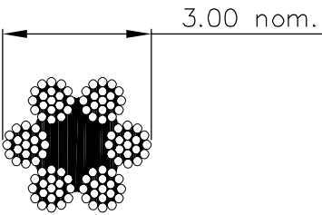
SCALE 10:1
